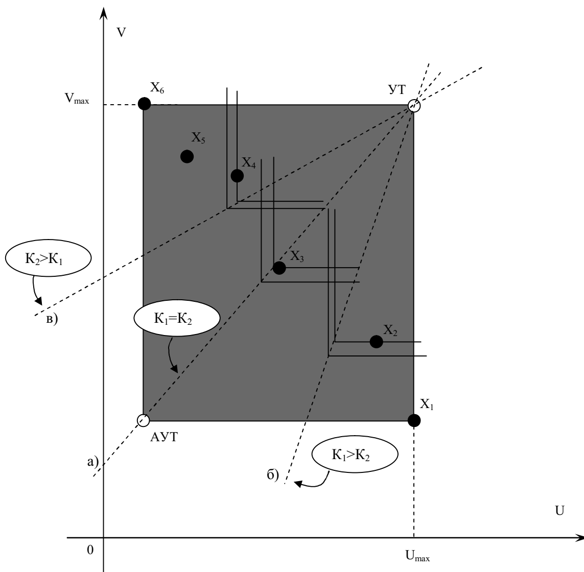
Рис. 5.7. Выбор в формате S_{GK(UT)} -критерия:
