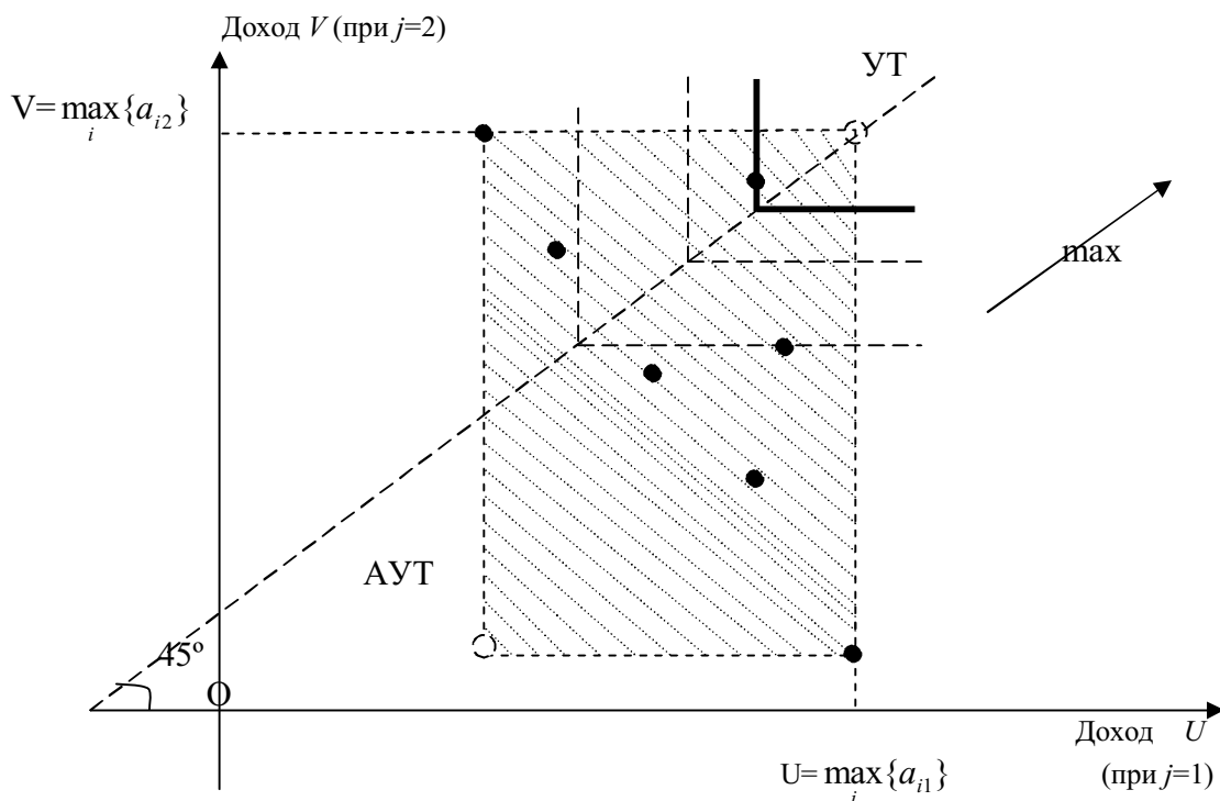
Рис.1.4. Линии уровня S -критерия:
