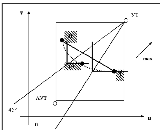
Рис. 8.1. Графическая интерпретация линий уровня S_{Gk(yT)} -критерия.
