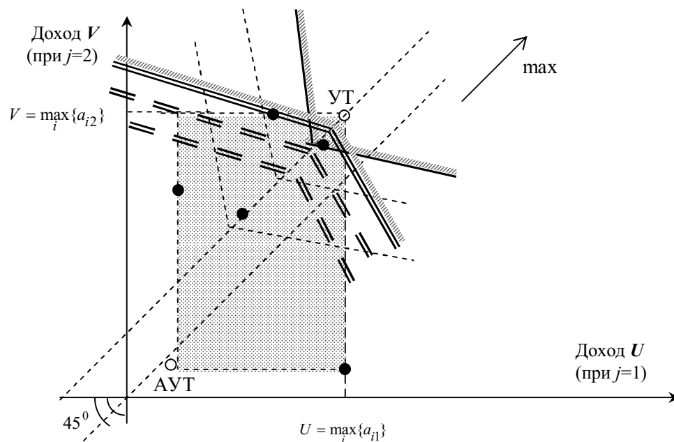
Рис. 4.2. Линии уровней для HW_{mod(VT)} -критерия:
