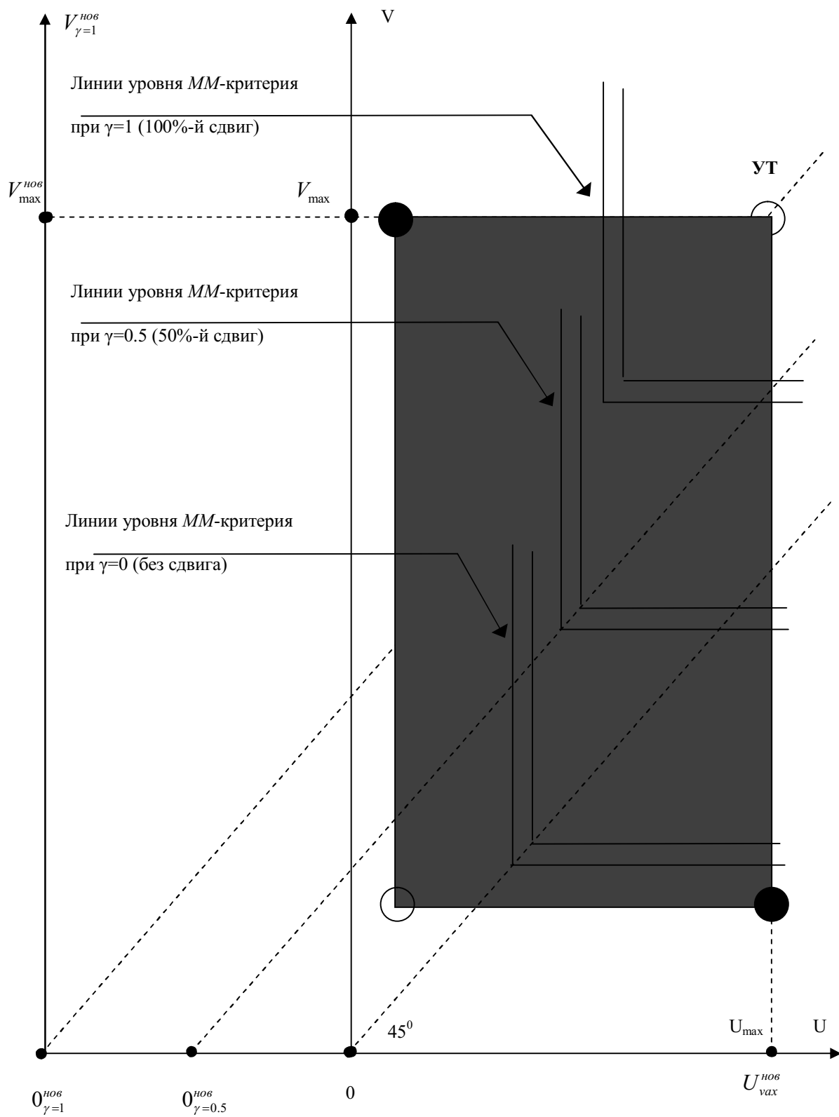
Рис. 6.1. Иллюстрация частичного сдвига линий уровня MM -критерия
