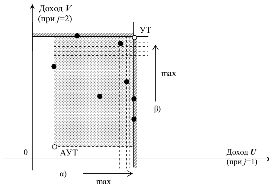
Рис. 2.56. Специфика выбора для критерия наиболее вероятного исхода.
