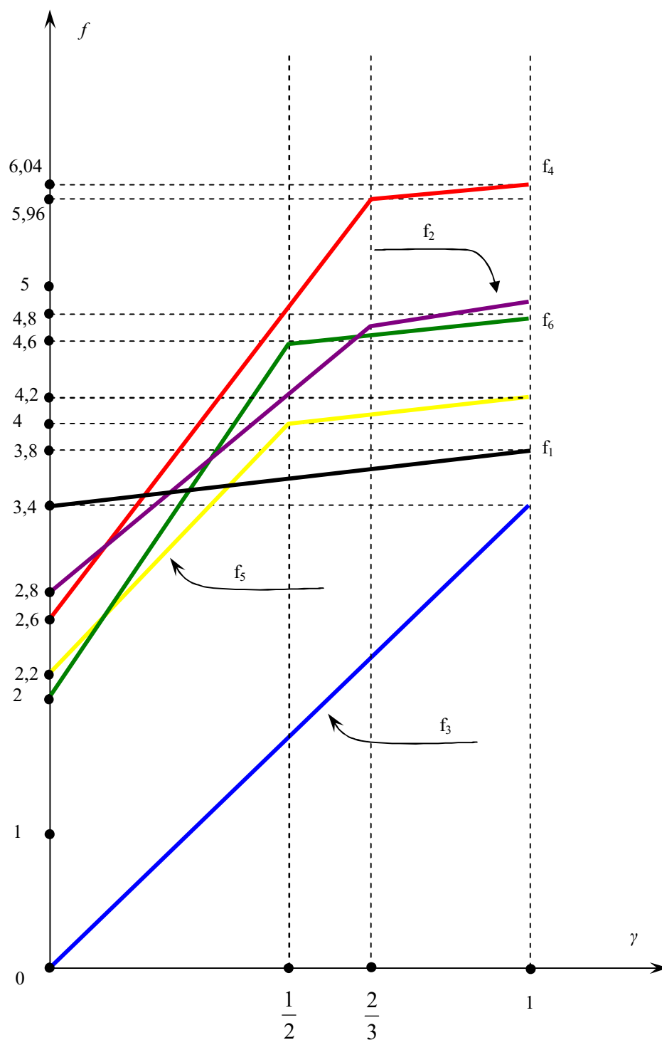
Рис. 6.6. Показатели альтернатив для NW_{\gamma(UT)} -критерия при c = 0,8 как функции f_i - f_6 переменного \gamma \in [0; 1] .
